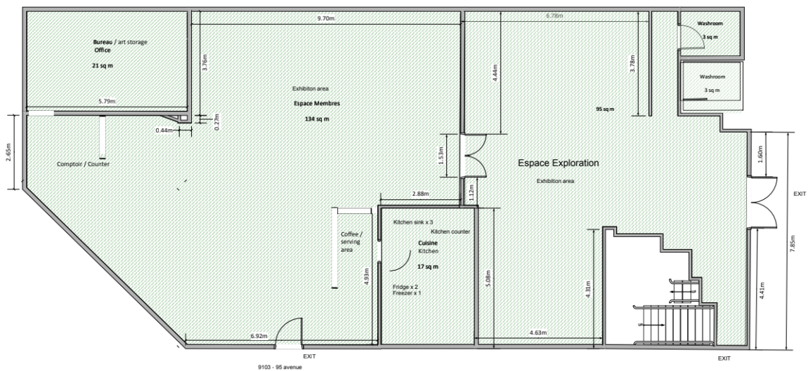
Plan d'Étage: CAVA
